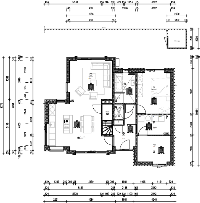
BEGANE GROND
