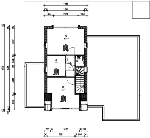
1E VERDIEPING
